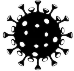
Coronavirus 2019-nCoV
